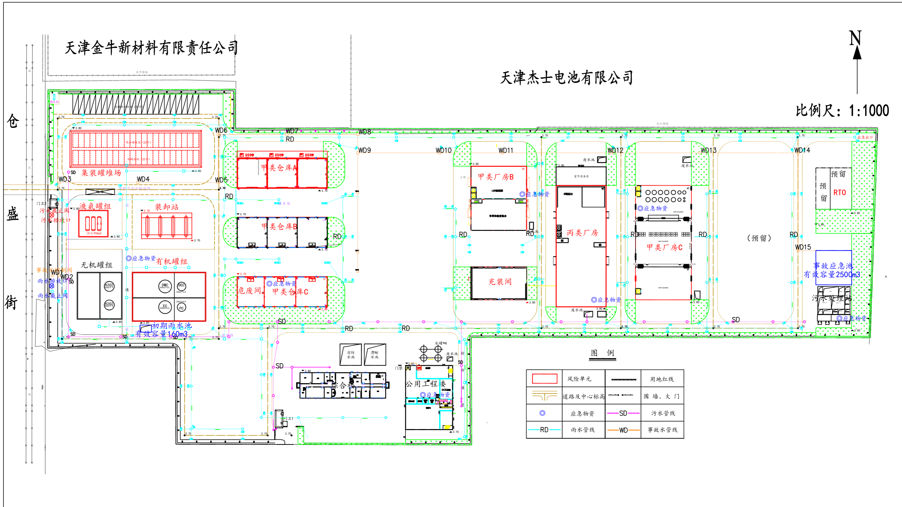
附图6 环境风险单元、应急物资和雨污水管网图
