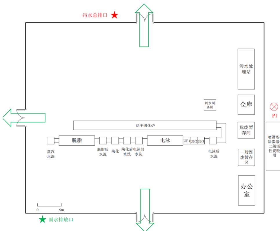
图 2.1-2 厂区紧急疏散图
