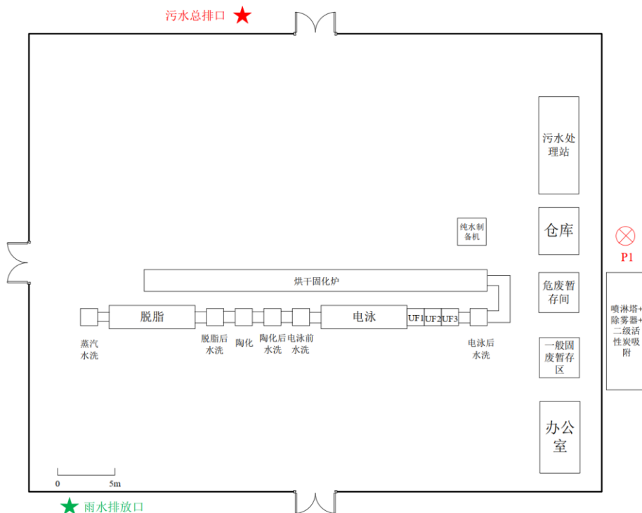
图 2.1-1 本公司平面布局图
